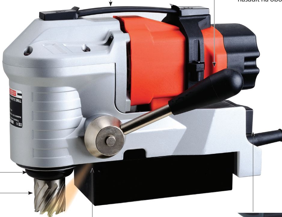
Kliku posuvu je možno nasadit na obou stranách
